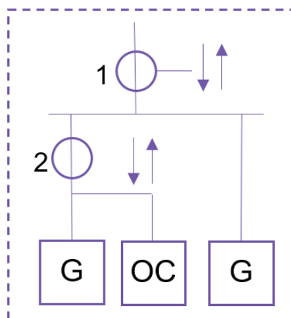
Figur 12. Mätare för energilagring som kan nettas mot annan produktion.
