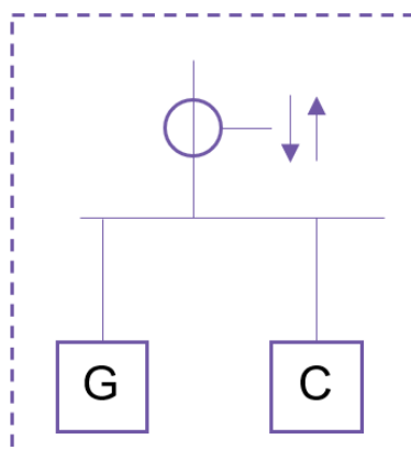
Figur 11. Mätare för energilagring som inte kan nettas mot produktion eller förbrukning.
