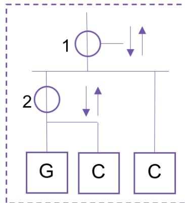
Figur 13. Mätare för energilagring som kan nettas mot annan förbrukning.
