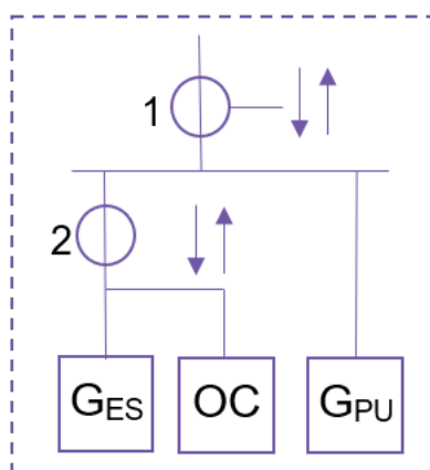
Figur 12. Ett exempel på en mätare för energilager som kan nettas mot annan produktion.
