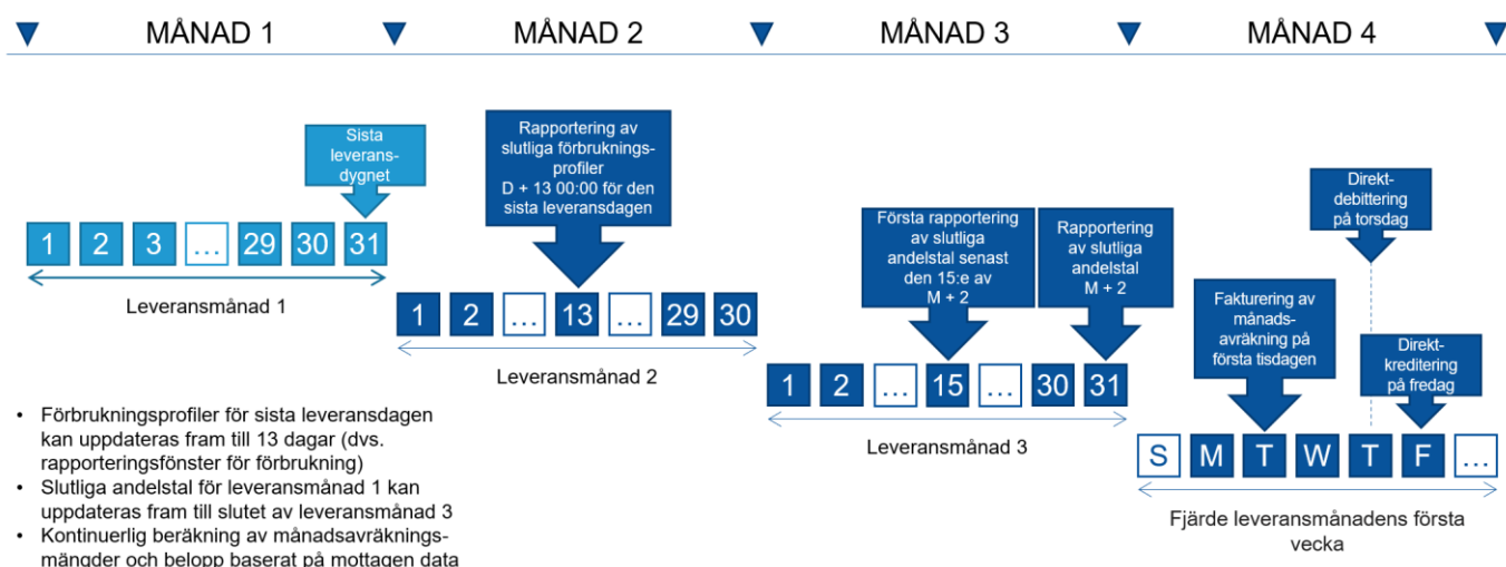
Figur 28. Schema för schablonavräkning, fakturerings och betalning.
