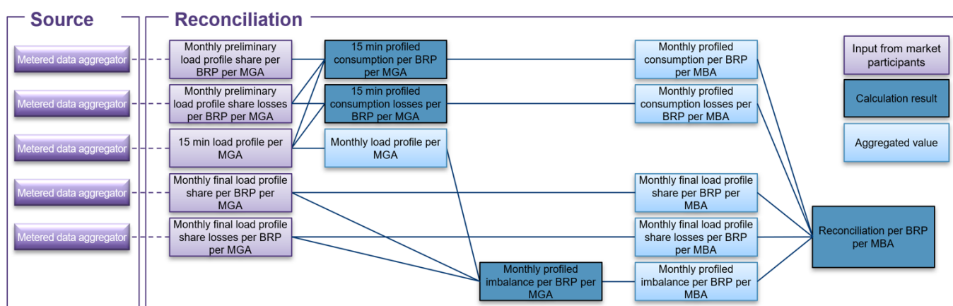
Figur 22. Beräkning av schablonavräkningen
