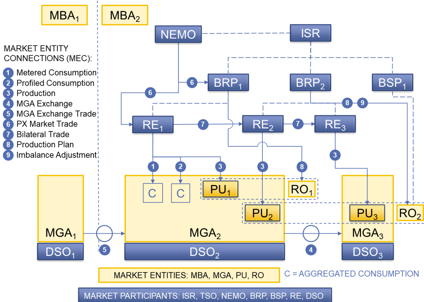
Figur 7. Exempel på delar som ingår i strukturen och deras inbördes förhållanden
