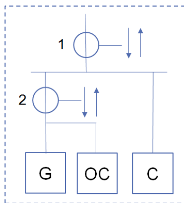
Figur 10. Mätare för produktion, egenförbrukning och förbrukning
