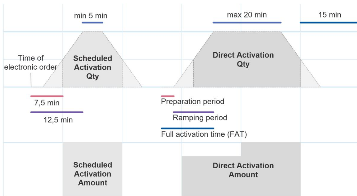
Figur 19. Volymrampning av mFRR-aktiveringar under tre eller fyra avräkningsperioder av obalanser (ISP)
