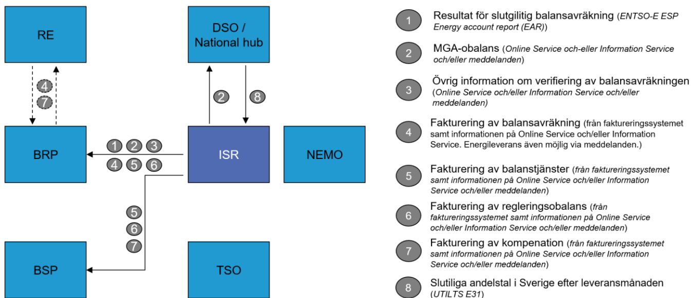
Figur 16. Rapportering efter avslutad balansavräkning (13 dagar).
