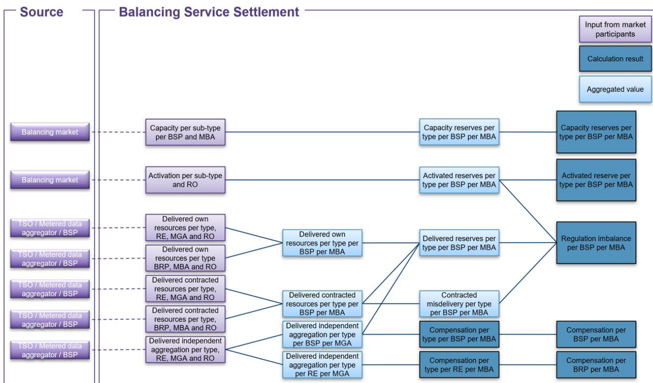
Figur 21. Beräkning av avräkning för balanstjänster.
