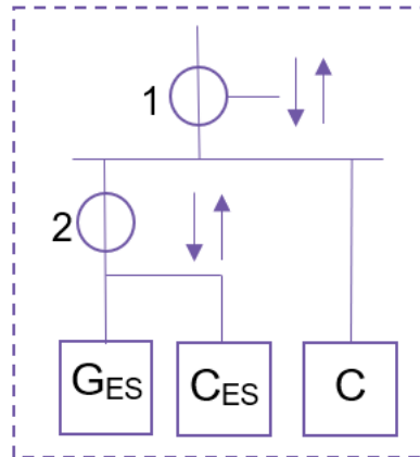
Figur 13. Ett exempel på en mätare för energilagring som kan nettas mot annan förbrukning.
