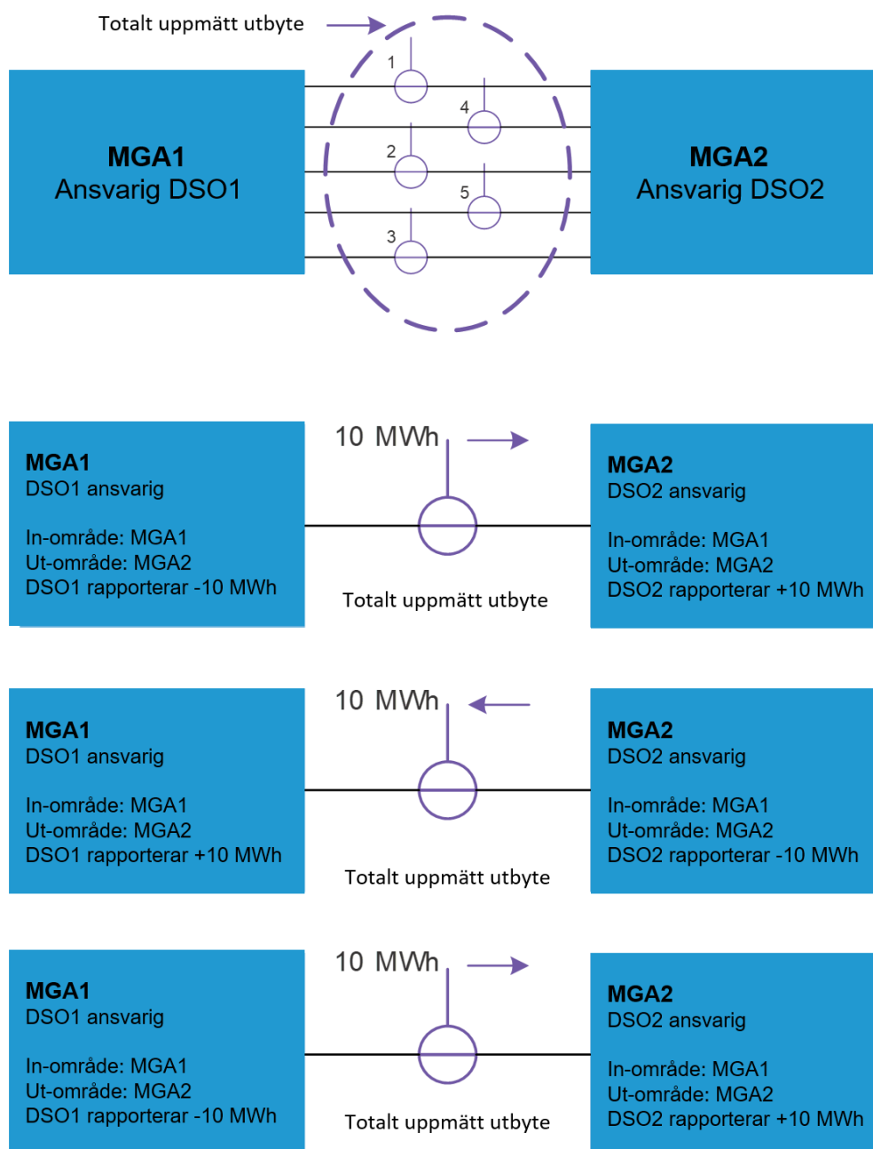
Figur 18. Exempel på rapportering av nätavräkningsområdesutbyte
