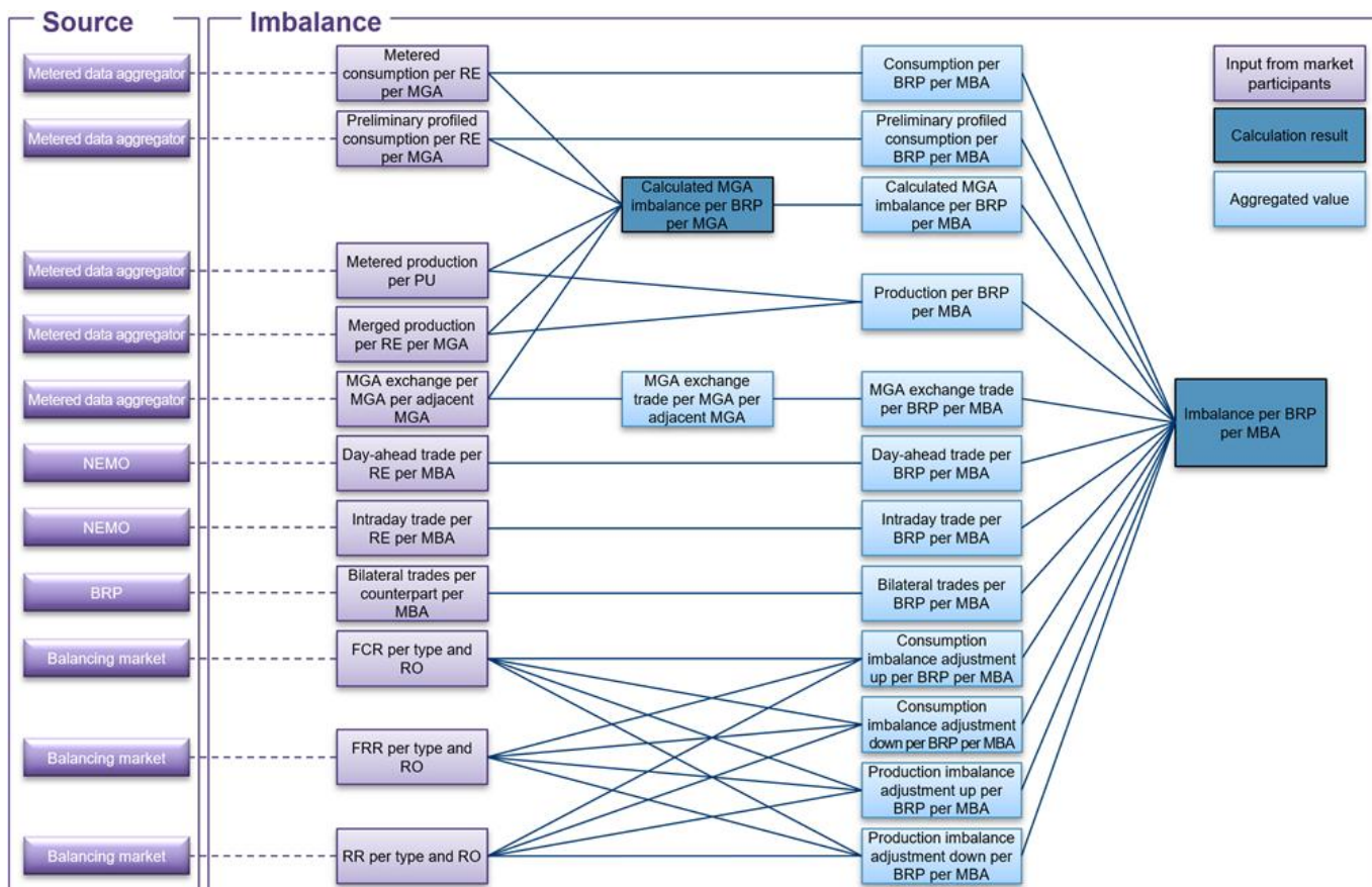
Figur 20. Beräkning av balansavräkning.
