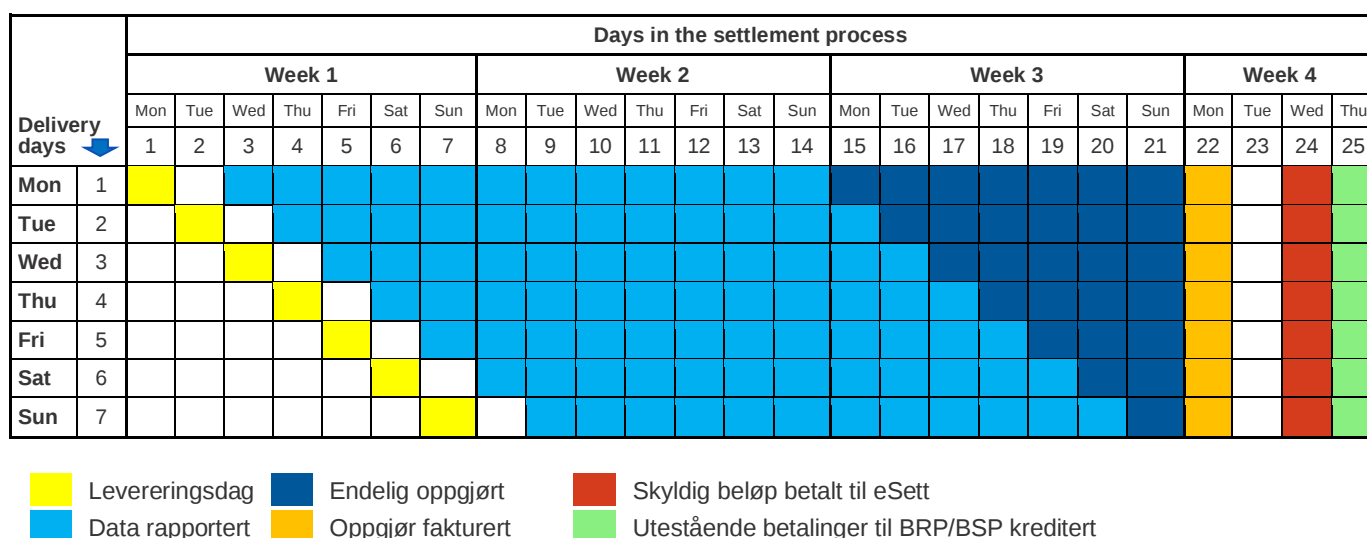
Figur 14 Tidsplan for oppgjør, fakturering og betaling
