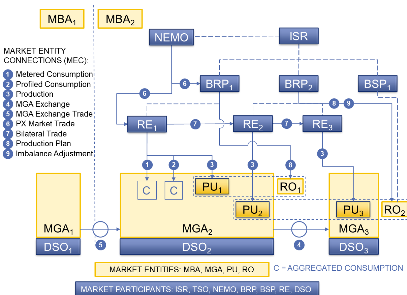
Figur 4 Eksempel på strukturelementer og deres forbindelser
